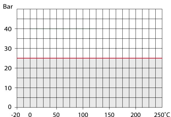
PN 25: Svejse × Svejse - DN 65 - 200
