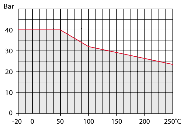
PN 40: Flange × Flange - DN 15 - 50
