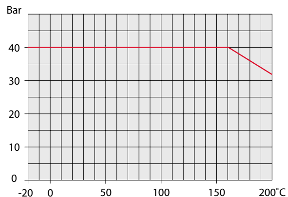
PN 40: Svejse × Svejse / Flange × Flange - DN 700 - 1000
