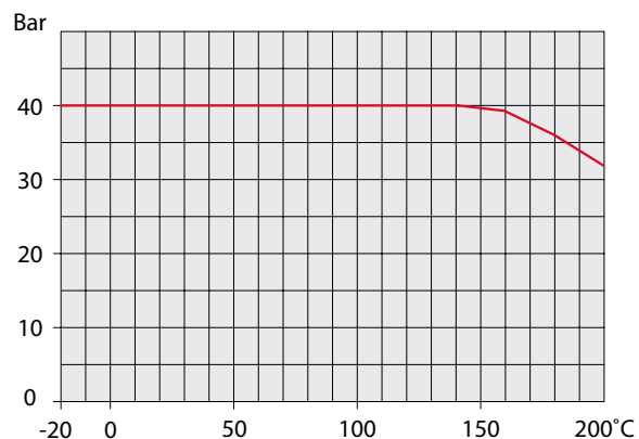
PN 40: Svejse × Svejse / Flange × Flange - DN150-600
