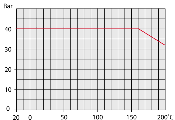
PN 40: Svejse x Svejse / Flange x Flange - DN 700 - 1000
